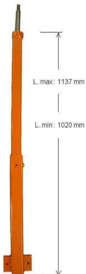
Dimensions de la potence de fixation
